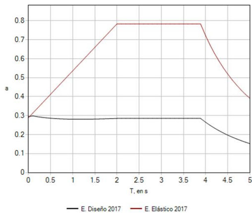
Figura 1. Espectro elástico sin modificar
